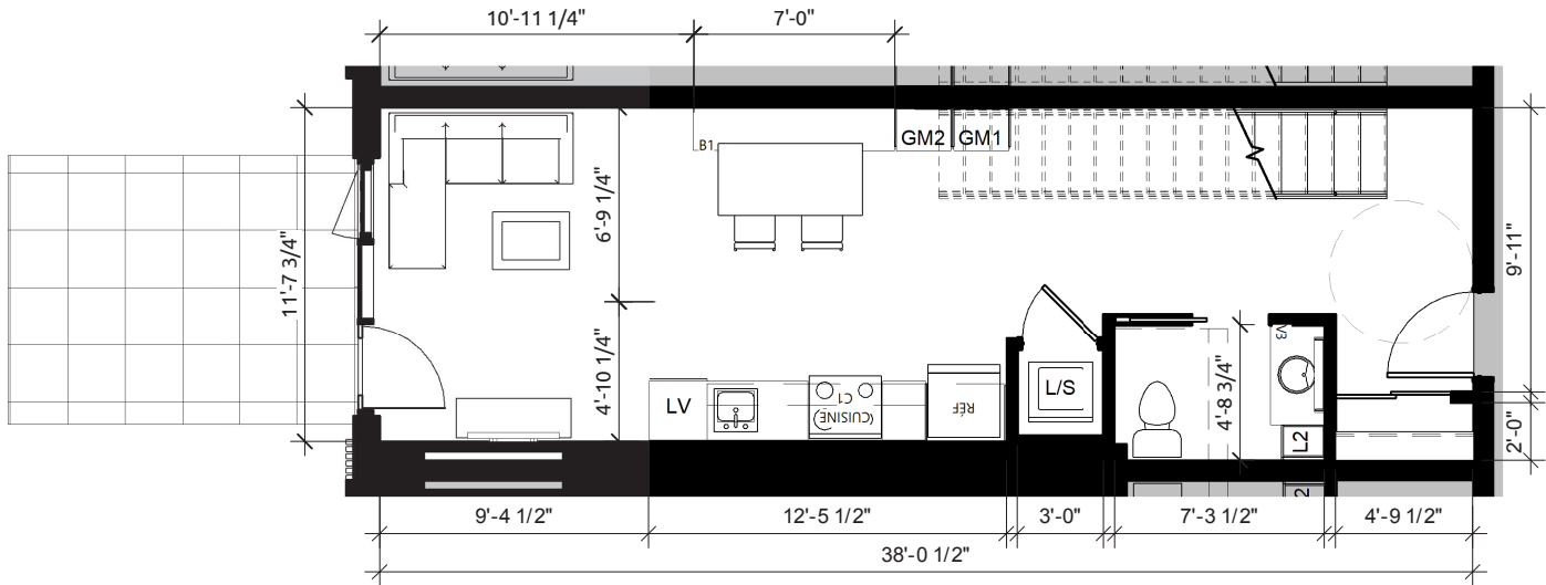
Niveau 01
